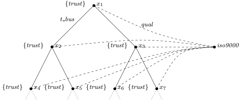
Fig. 1. Forest-Model
